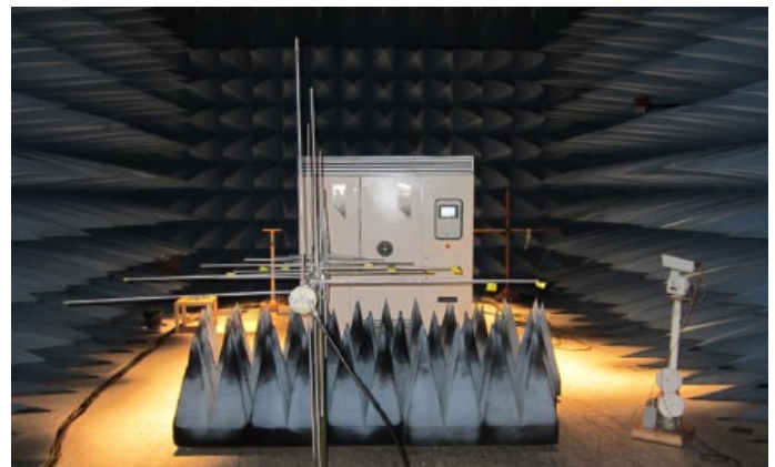
Inversores PVWD en la cámara anecoica para medir su inmunidad electromagnética
